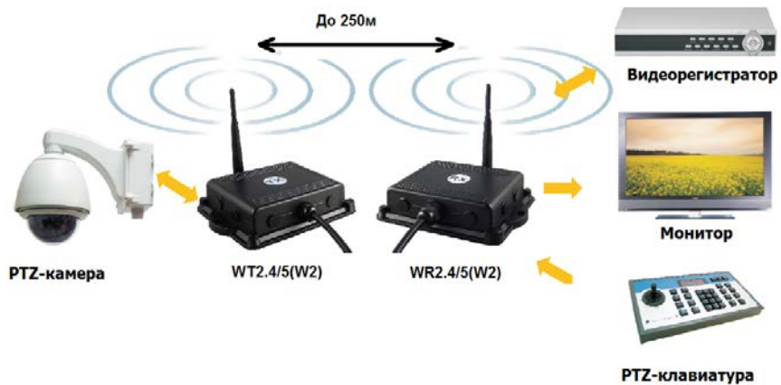
Рис.4 Схема подключения передатчика WT2.4/5(W2) и приёмника WR2.4/5(W2).
