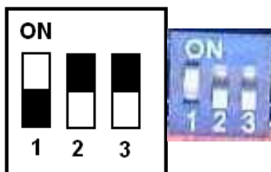
Рис.9 Внешний вид DIP-переключателей.
