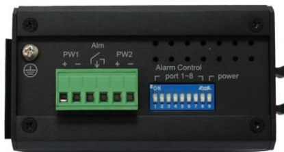
Рис.1 Внешний вид коммутатора SF-30602/1
