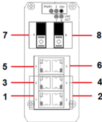
Рис.3 Порты коммутатора SF-30602/1
