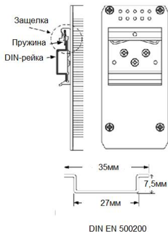
Рис.7 Монтаж коммутатора SF-30602/I на DIN-рейку.
