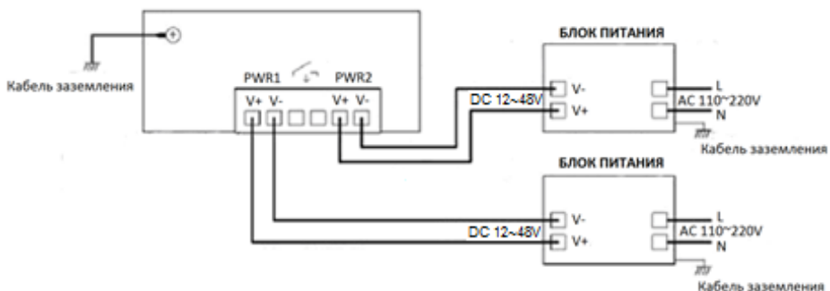
Рис.8 Схема подключения блоков питания к клеммной колодке коммутатора SF-30602/1
