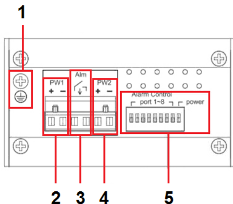
Рис.4 Клеммная колодка и Dip-переключатели коммутатора SF-30602/1
