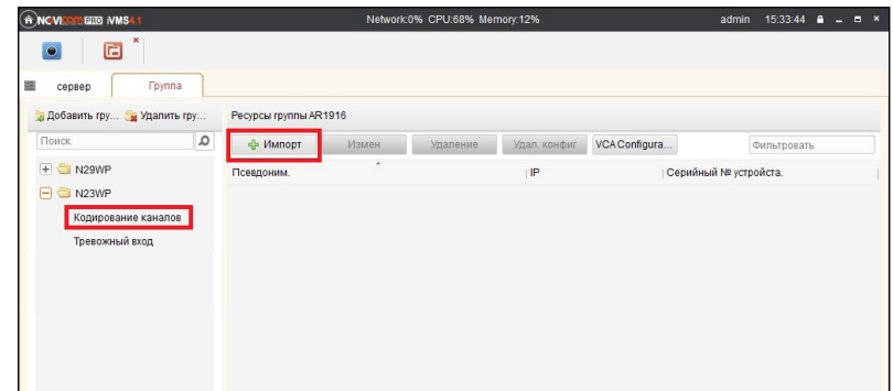
Рис.31 Импорт камеры.
