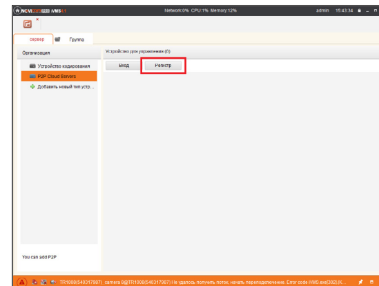
Рис.26 Регистрация.
