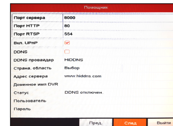
Рис. 14 Настройка портов.
