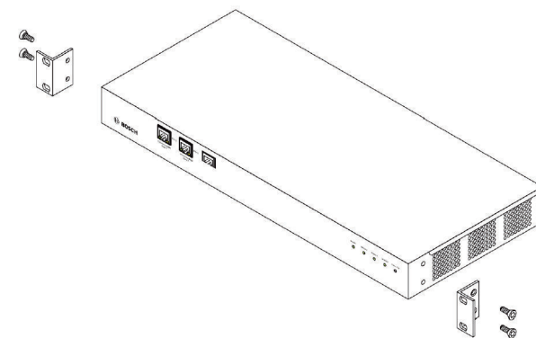
Принадлежности для монтажа VIP X1600 XF в стойке
