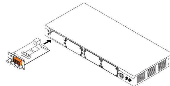
Сборка модуля VIP X1600 XF
