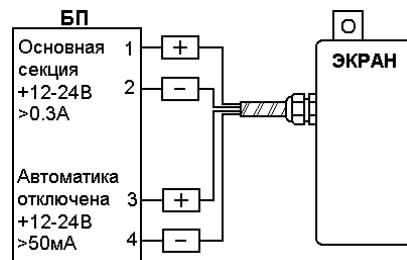
Рисунок 3. Подключение оповещателей ЭКРАН-С/СЗ с дополнительной секцией.
