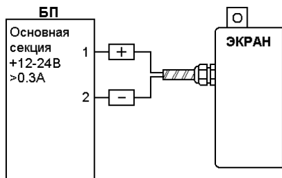
Рисунок 2. Подключение оповещателей ЭКРАН-С/СЗ/СУ.
