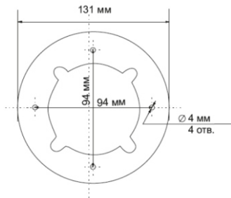
Рис.3 Крепежная платформа
