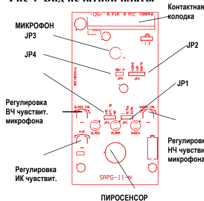
Рис 4 Вид печатной платы
