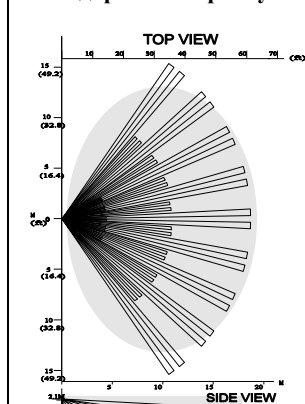
Рис 5 Диаграмма направленности стандартной широкоугольной линзы
