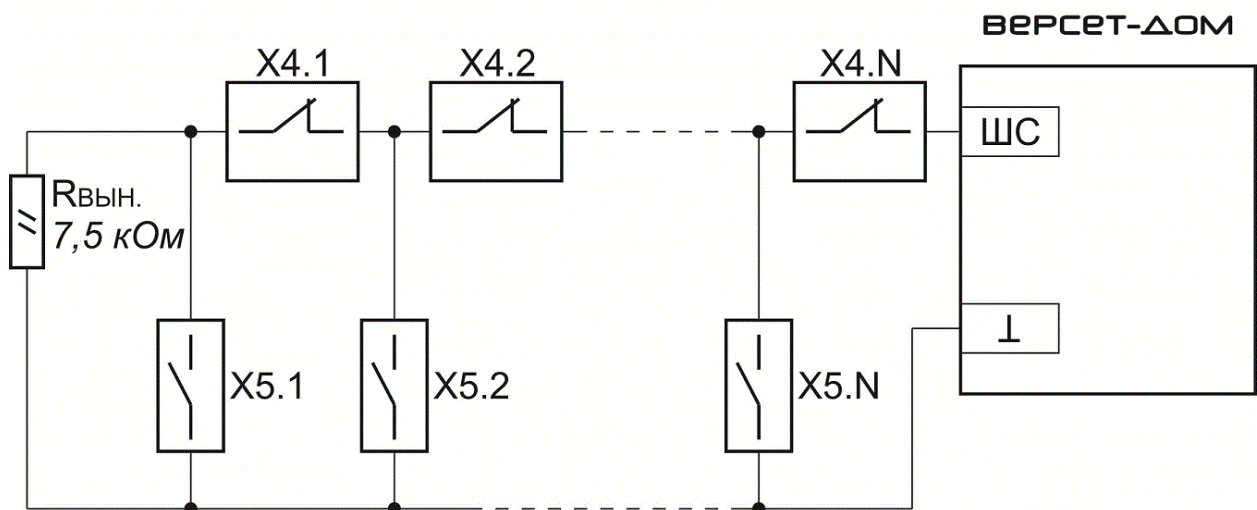
Рис.14. Схема подключения охранных извещателей к охранным ШС. X4 - извещатели охранные с нормально замкнутыми контактами X5 - извещатели охранные с нормально разомкнутыми контактами
