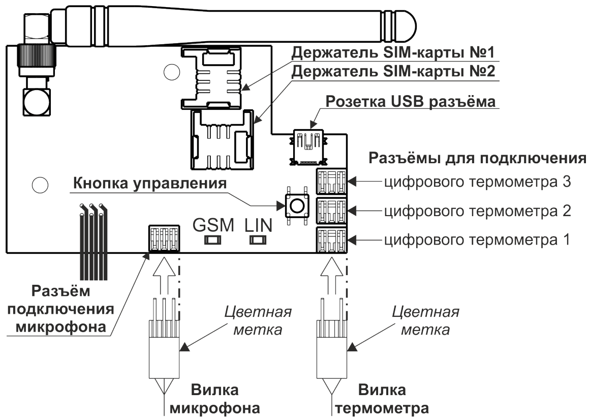
Рис.24. Вид платы коммутатора прибора.
