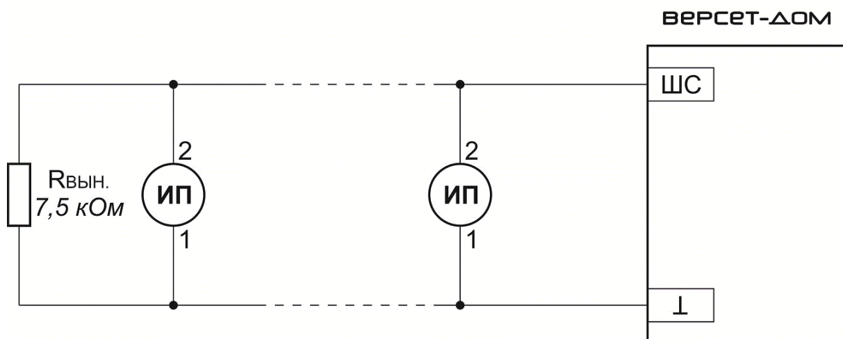
Рис 21. Схема подключения пожарных тепловых извещателей ИП101 – 1А – А1 к пожарному ШС. Однороговой режим работы.
