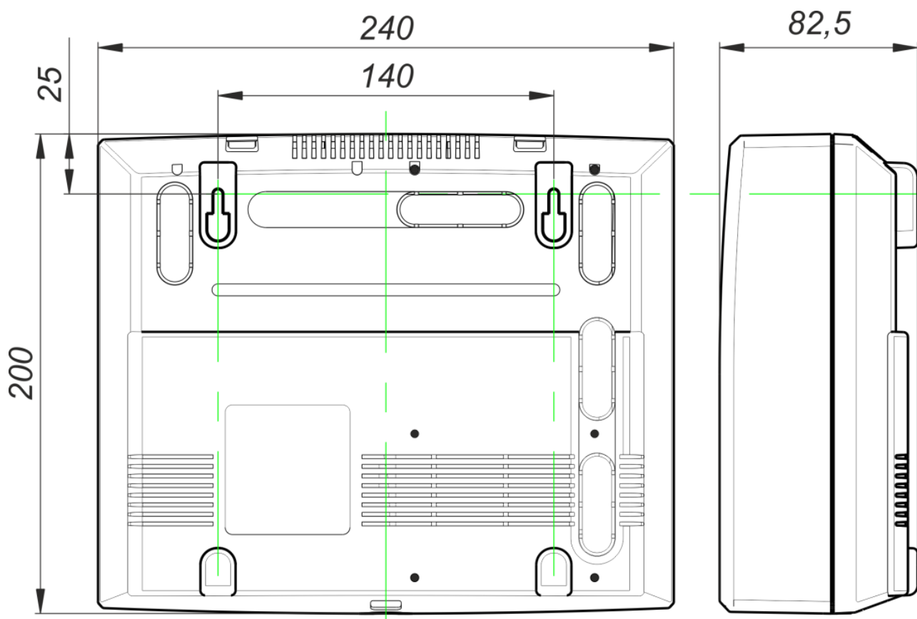
Рис.22. Габаритные и установочные размеры прибора ВЕРСЕТ 2(4,8) GSM ВЕРСЕТ - ДОМ.
