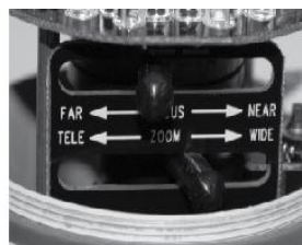
Запатентованная система настройки объектива
