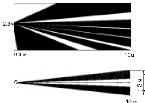
Рис. 1. Диаграмма зоны обнаружения
