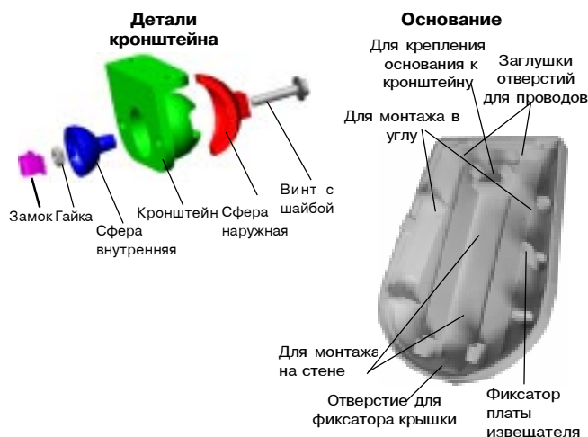
Крепление кронштейна на стене
