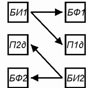
Пример 4-х лучевой ИК шторы
