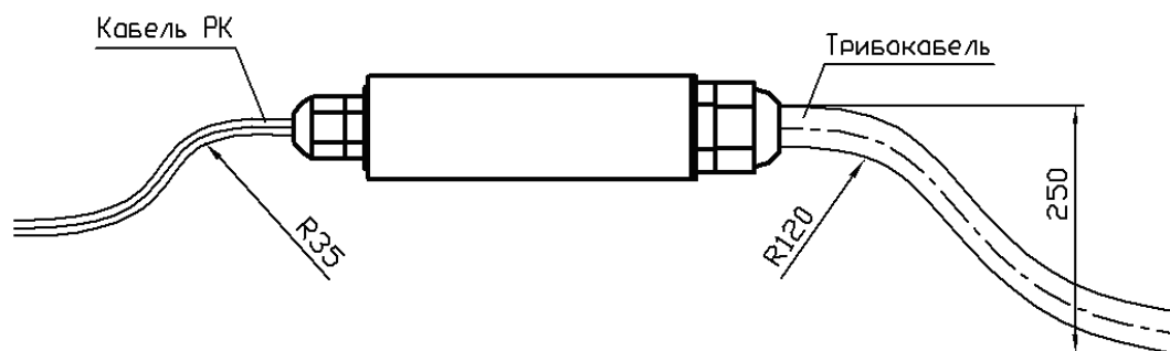
Рисунок А.12.1 – Пример установки муфты переходной
