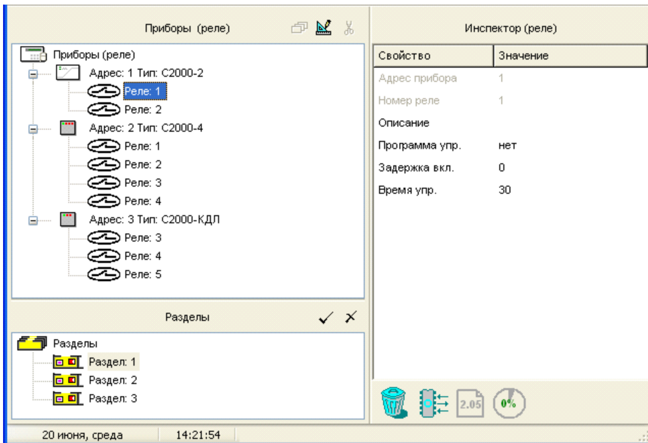
Рисунок 23. Страниц «Реле» с группировкой по приборам
