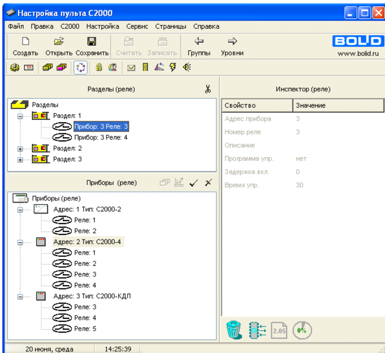
Рисунок 24. Страница «Реле» с группировкой по разделам
