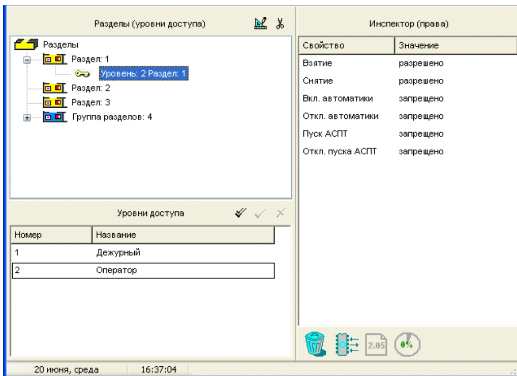
Рисунок 26. Страница «Уровни доступа» с группировкой по разделам
