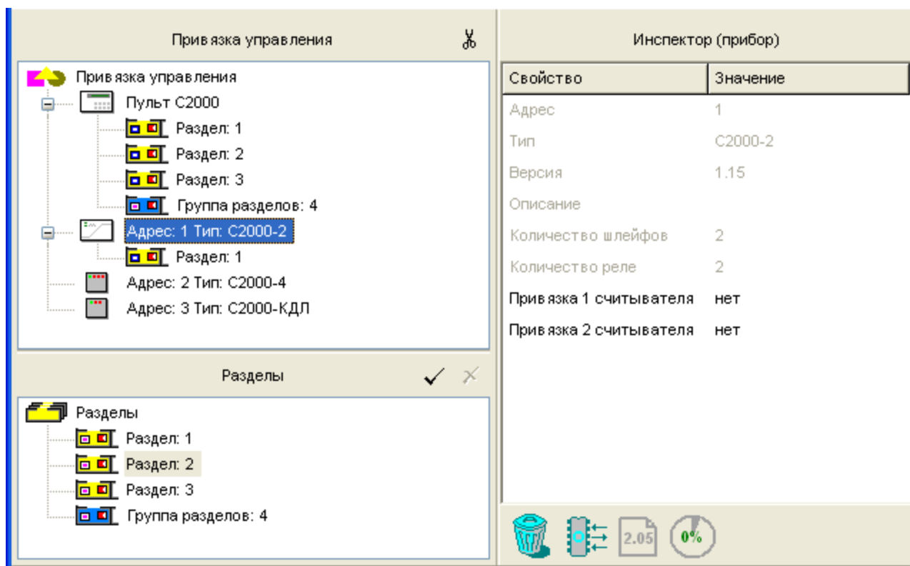
Рисунок 37 Страница «Привязка управления»
