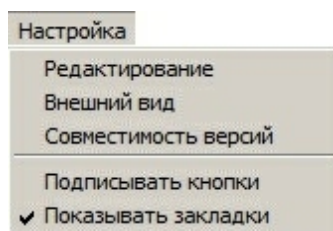
Рисунок 6. Меню «Настройка»
