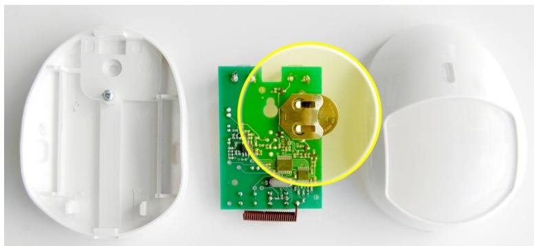
Рис. 8.2. Установка резервного элемента питания в радиоизвещатель Фотон-19-РК
