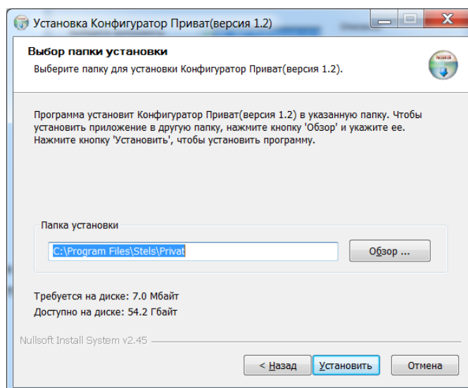
Рис. 5.2. Выбор пути
