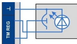
Рис. 12.2. Подключение считывателя Touch Memory со светодиодным индикатором
