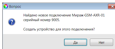
Рис. 5.11. Окно Вопрос
