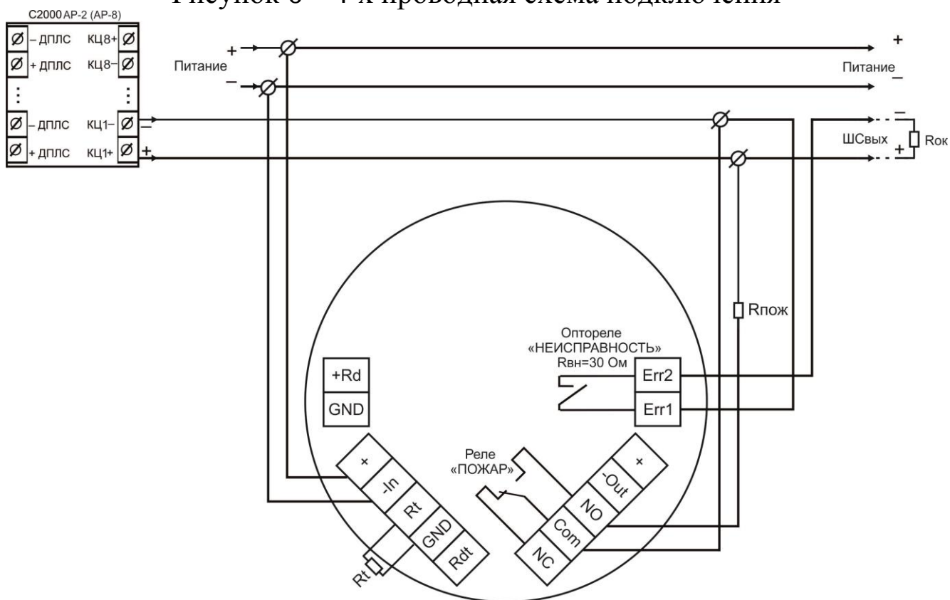
Рисунок 6 – 4-х проводная схема подключения
