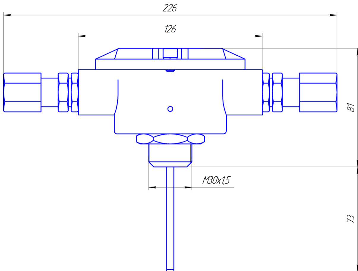
Рис. 1 – Извещатель пожарный тепловой ИП 101-СпектронТ-Р
