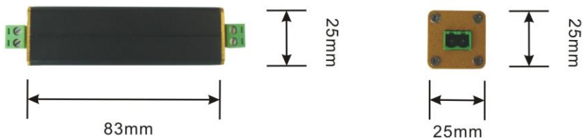
Рис.2 Габаритные размеры SP-IP/100
