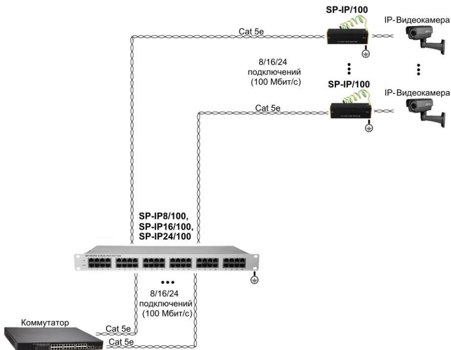
Рис.3 Подключение SP-IP/100
