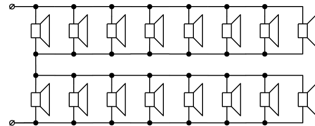
Подключение шестнадцати акустических оповещателей Zн=8 Ом, Pн=3Вт; Pвых≈1,5 Вт/оповещатель – рис.4
