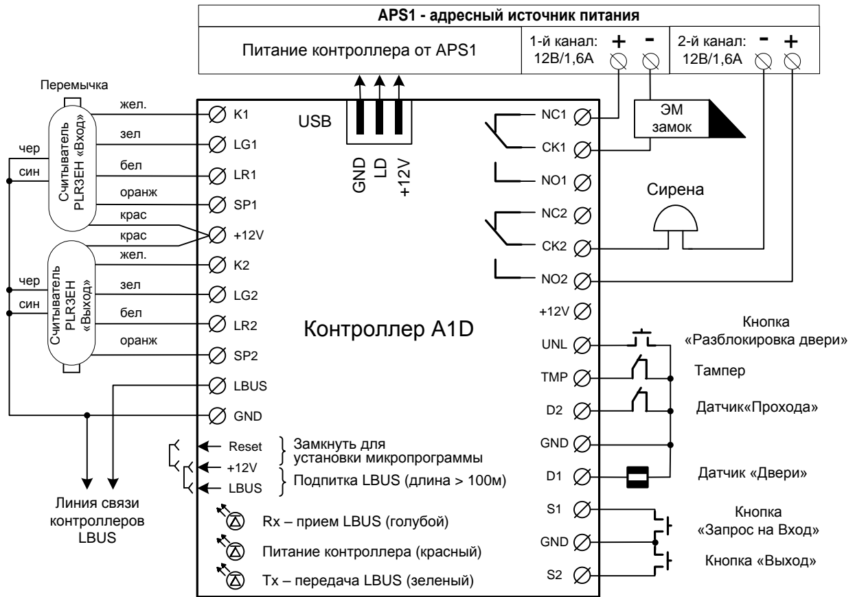
Рисунок 2 Схема подключения
