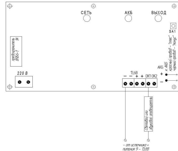
Рисунок 1 – Схема подключения «Импульс-1, 2, 3»
