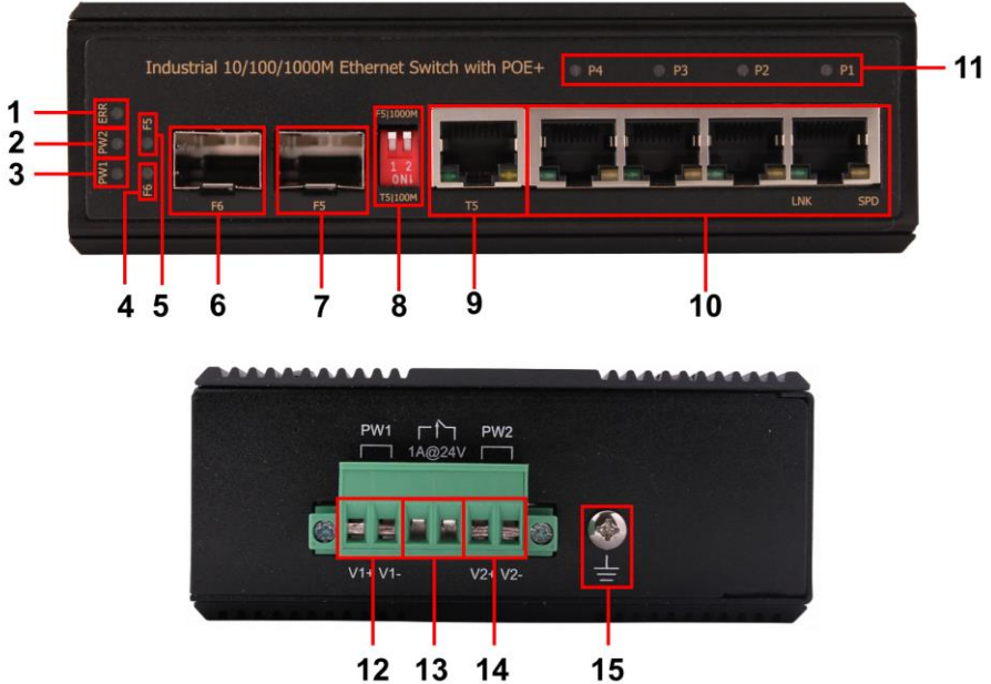
Рис. 3 Разъемы, DIP-переключатели и индикаторы коммутатора SW-80412/IC(Booster)
