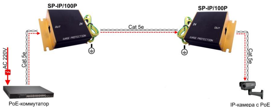
Рис.3 Подключение SP-IP/100P
