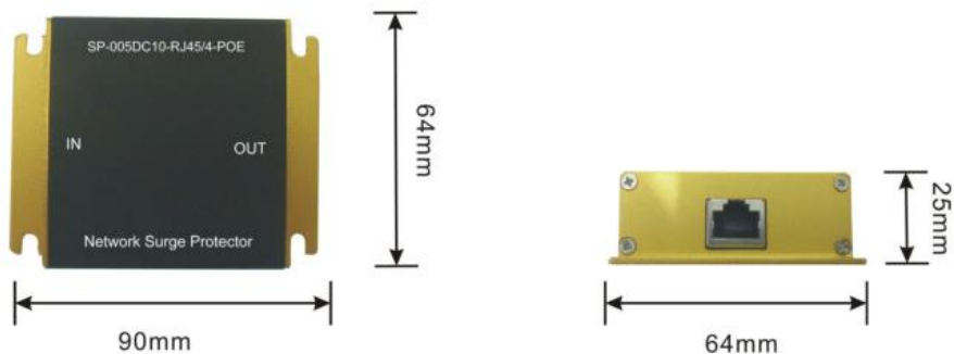
Рис.2 Габаритные размеры SP-IP/100P
