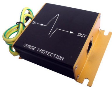
Рис.1 Внешний вид SP-IP/100P
