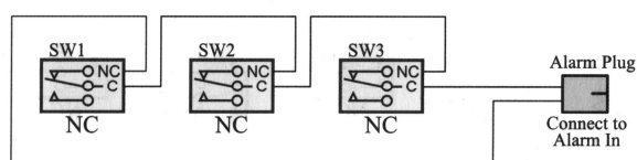
Рис.13 Последовательное подключение тревожных датчиков нормально-замкнутого типа
