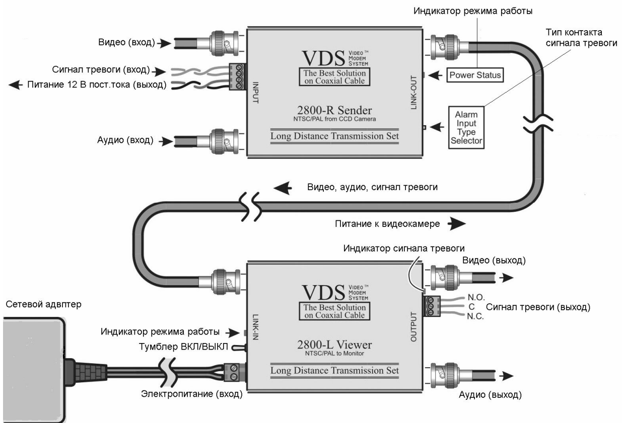
Рис.4 Структурная схема подключения VDS 2800
