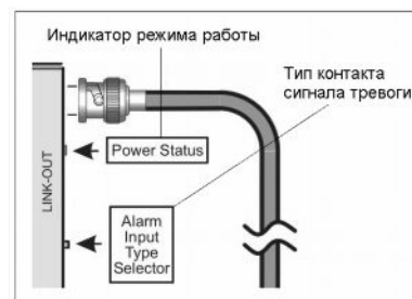
Рис.6 Подключение соединительного кабеля
