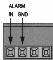
Рис.11 Клеммник для подключения тревожных датчиков
