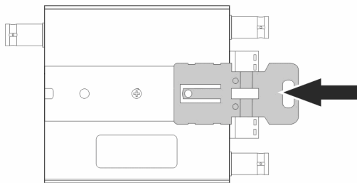
Рис.2.2 Монтаж крепления
