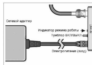
Рис.7 Подключение соединительного кабеля
