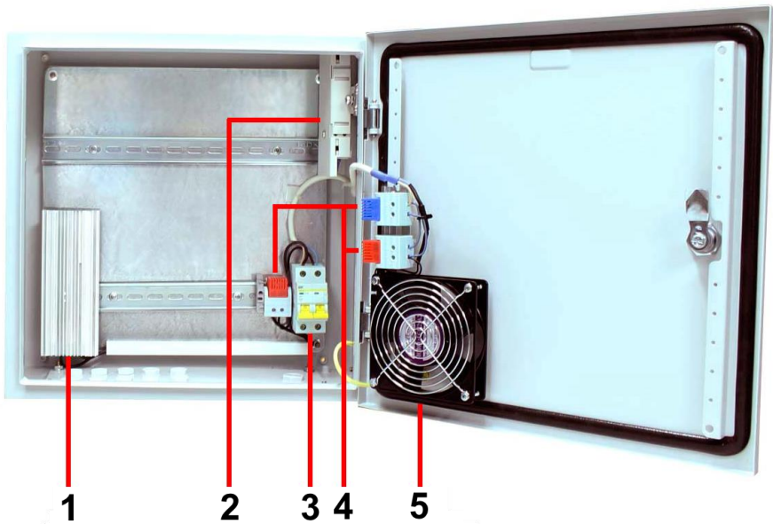
Рис.6 Уличная станция OS-44T1 с термостабилизацией, внутренние элементы
