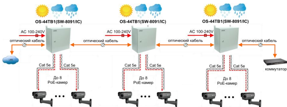
Рис.18 Типовая схема подключения уличных коммутаторов на примере модели OS-44TB1(SW-8091/IC)
