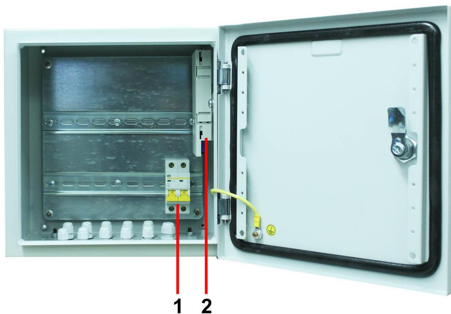
Рис.10 Уличная станция OS-331, внутренние элементы
