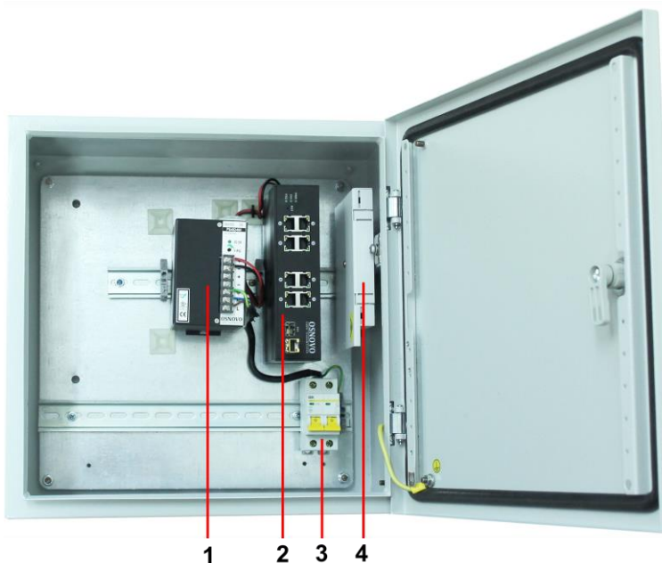
Рис.5 Уличный коммутатор OS-441 (SW-8091/IC), внутренние элементы
