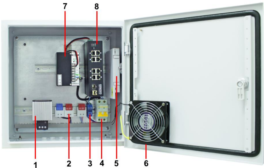
Рис.7 Уличный коммутатор OS-44T1(SW-8091/IC) с термостабилизацией, внутренние элементы
