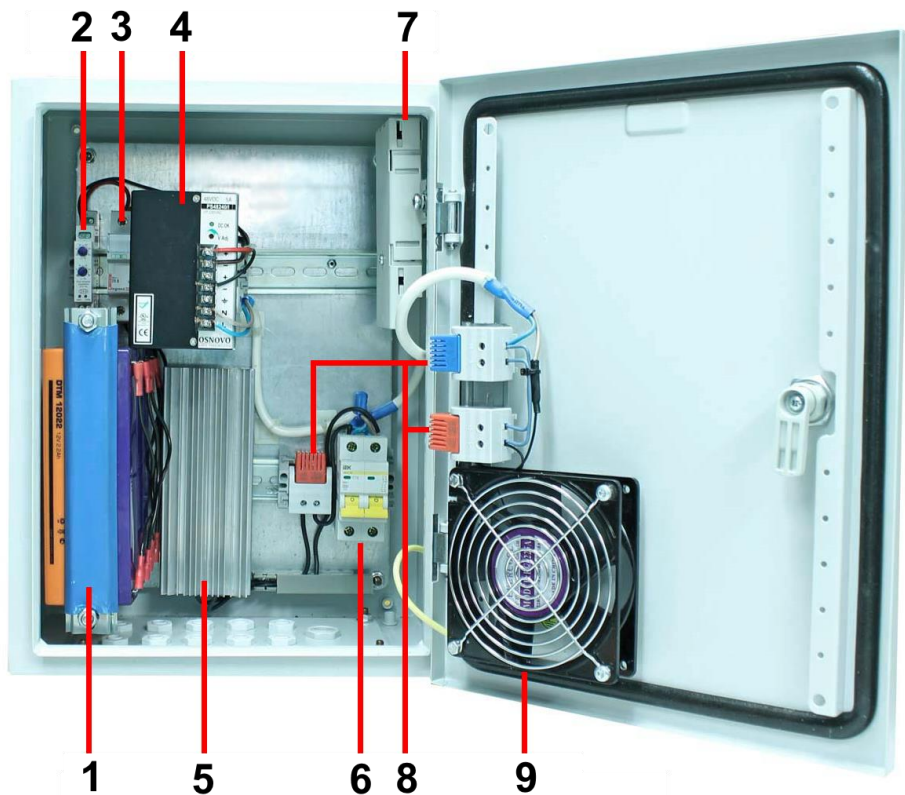
Рис.16 Уличная станция OS-34TB1 с термостабилизацией и системой резервного питания, внутренние элементы
