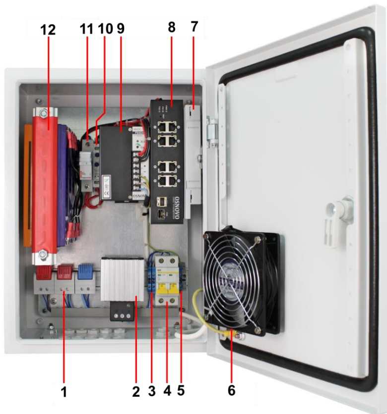
Рис.17 Уличный коммутатор OS-34TB1(SW-8091/IC) с термостабилизацией и системой резервного питания, внутренние элементы
