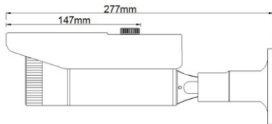
Рис.1 Вид сбоку
