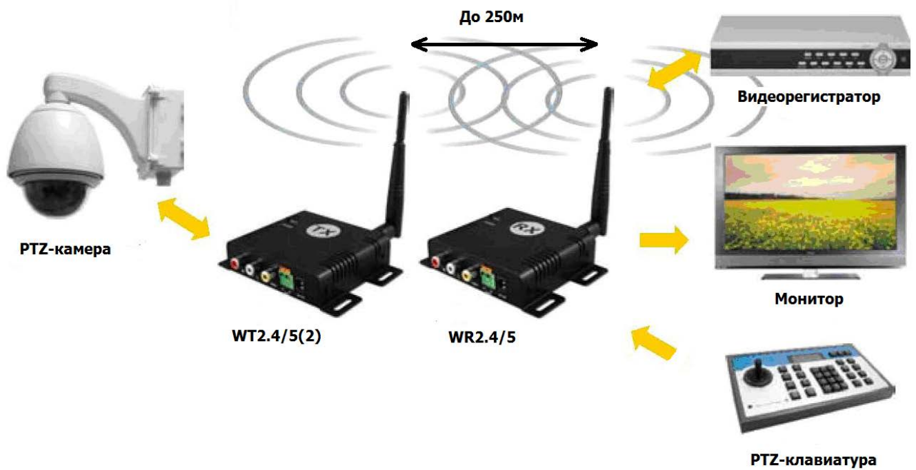
Рис.4 Схема подключения передатчика WT2.4/5(2) и приёмника WR2.4/5.
