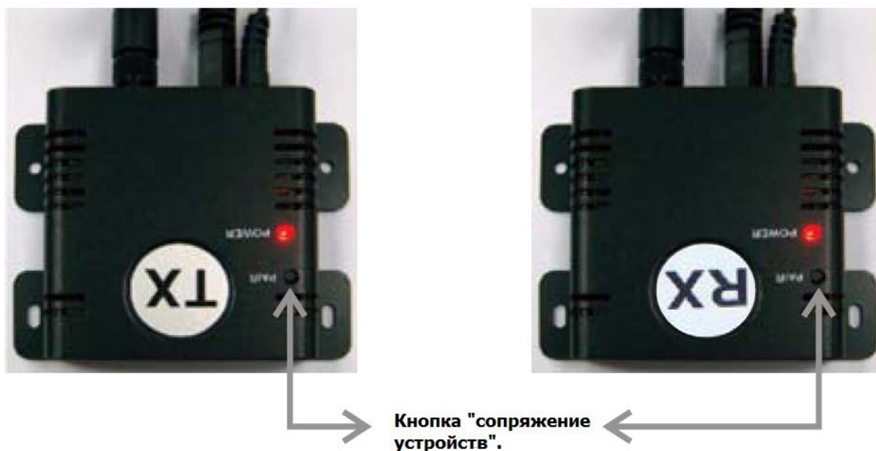
Рис.10 Сопряжение передатчика и приёмника.
