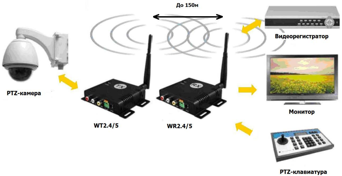
Рис.3 Схема подключения передатчика WT2.4/5 и приёмника WR2.4/5.
