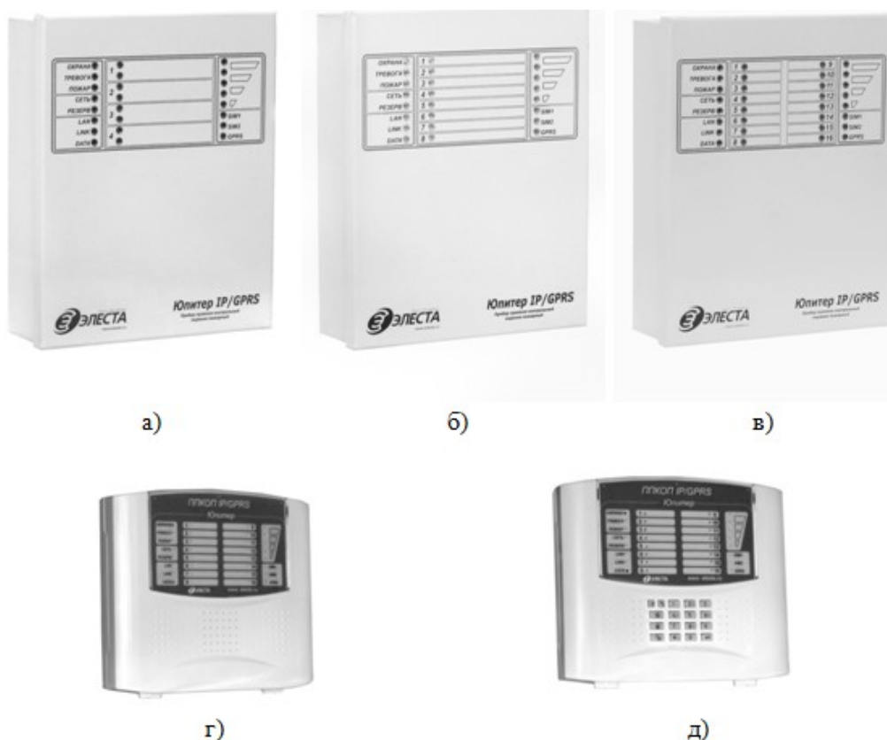
Рисунок 2.1. Внешний вид прибора ППКОП «Юпитер IP/GPRS» в различных вариантах исполнения: а) металлический корпус, четыре шлейфа, б) металлический корпус, восемь шлейфов, в) металлический корпус, 16 шлейфов, г) пластиковый корпус без встроенной клавиатуры, д) пластиковый корпус со встроенной клавиатурой
