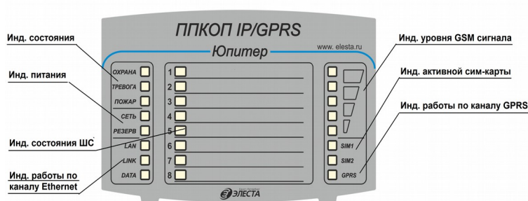
Рисунок 2.3. Панель индикации ППКОП «Юпитер IP/GPRS»
