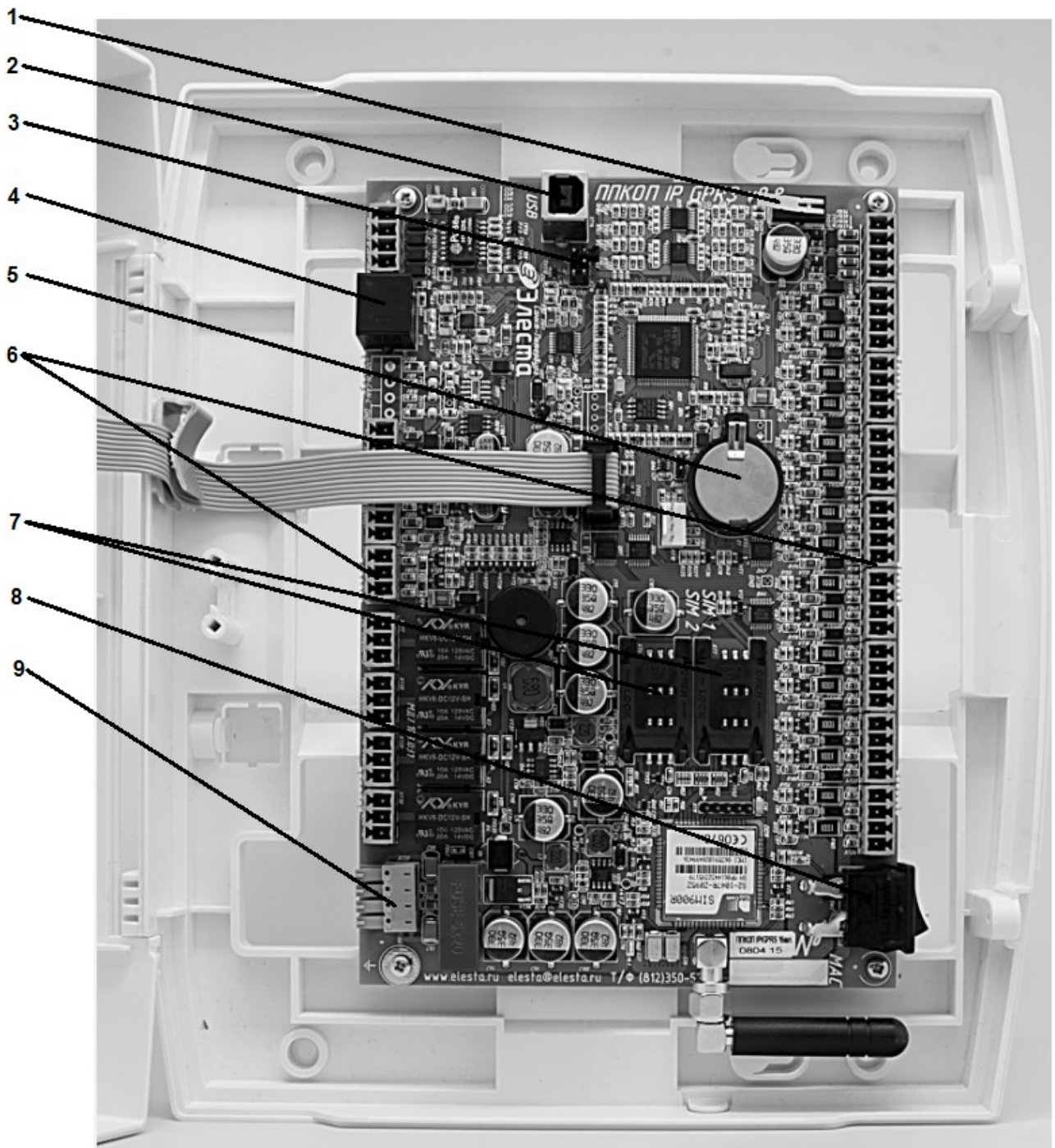
Рисунок 2.2. Вид прибора с открытой крышкой
