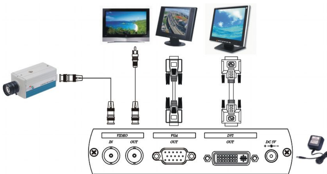
Рис.2 Структурная схема подключения
