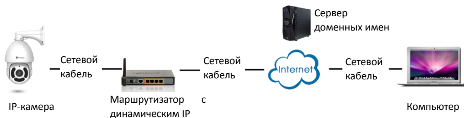
Рис. 2-2. Подключение сетевой камеры через маршрутизатор, используя динамический IP-адрес.
