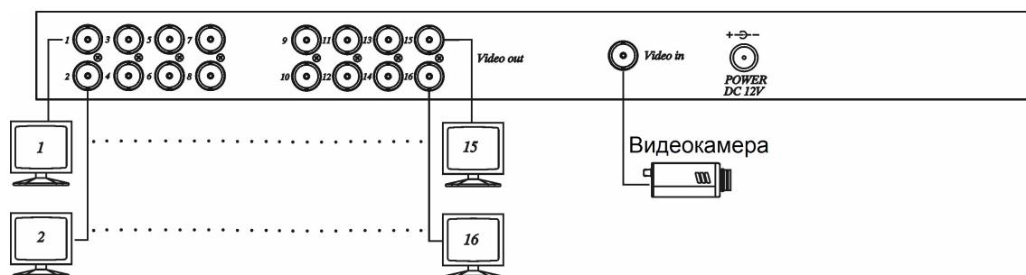
Рис.2 Структурная схема подключения
