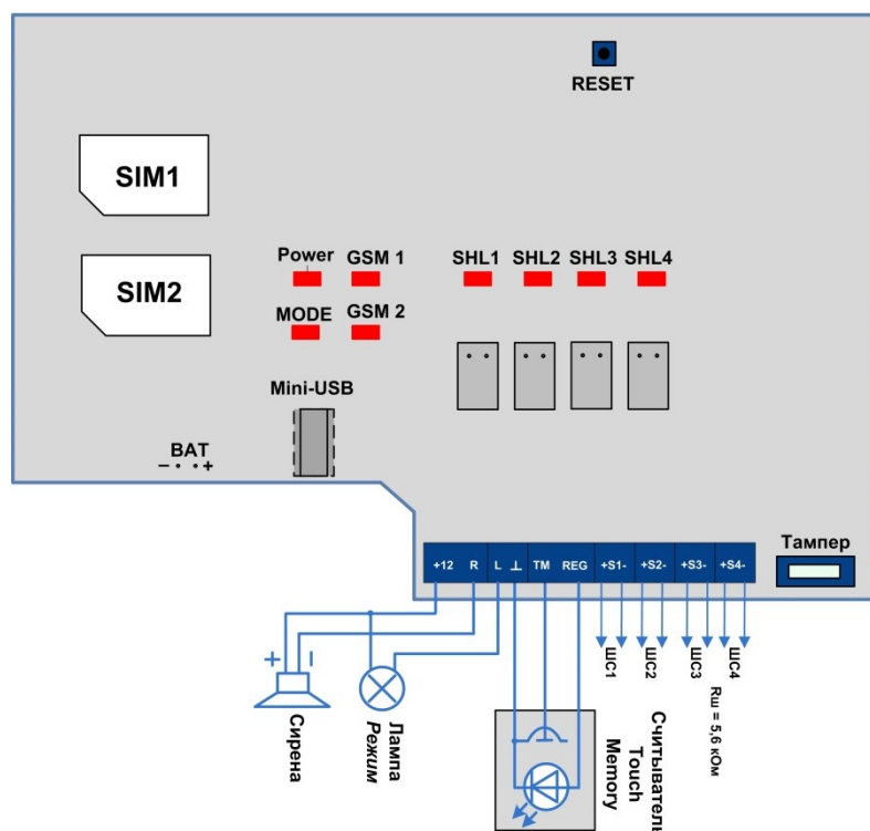
Рис. 10.2. Схема внешних подключений
