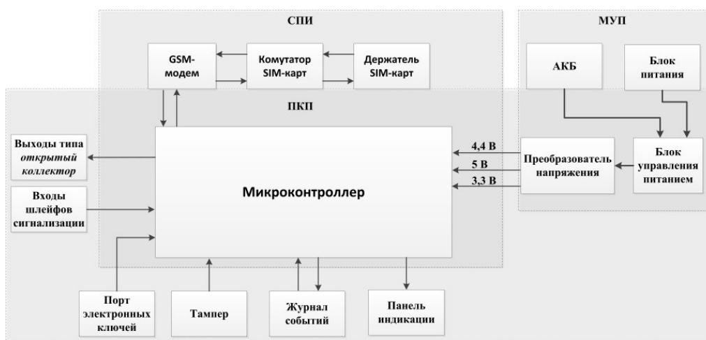
Рис. 3.1. Функциональная схема контроллера
