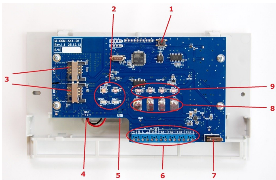
Рис. 10.1. Вид контроллера со снятой крышкой
