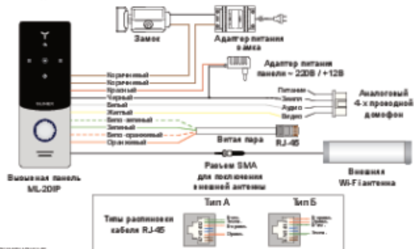
Схема 1. Подключение питания и звонка к панели ML-201P.
