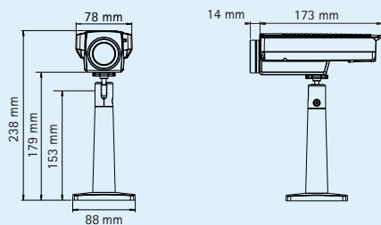
Размеры: Сетевая камера AXIS Q190
