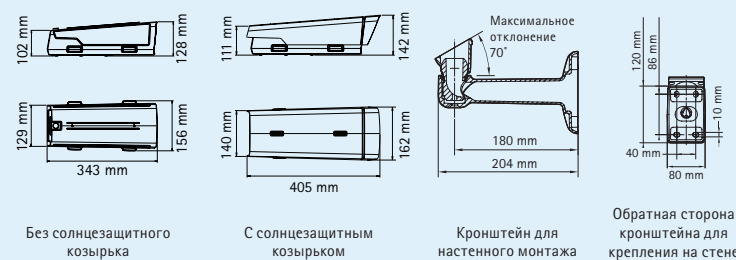
Размеры: Сетевая камера AXIS Q190-E с кронштейном для крепления на стене и внутренним каналом для кабеля
